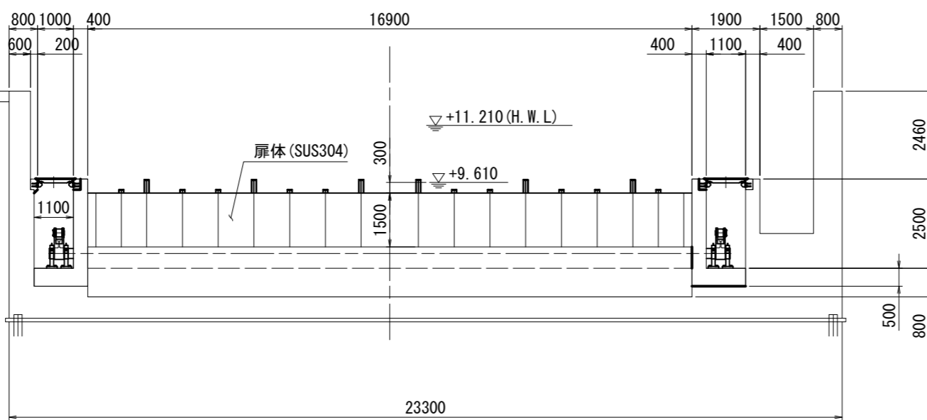
正面図 (S=1:100)
