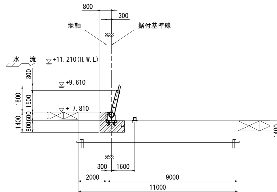
断面図 (S=1:100)
