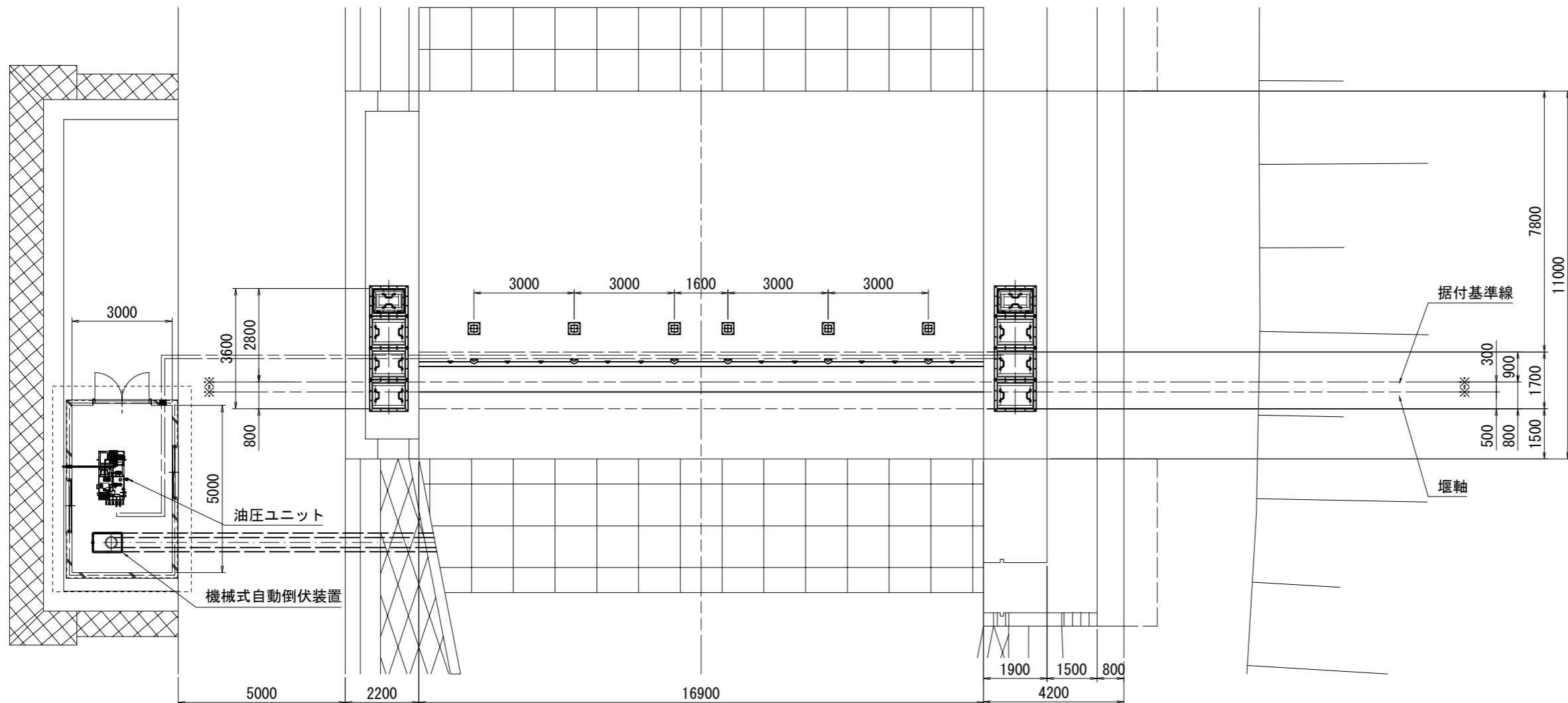
平面図 (S=1:100)
